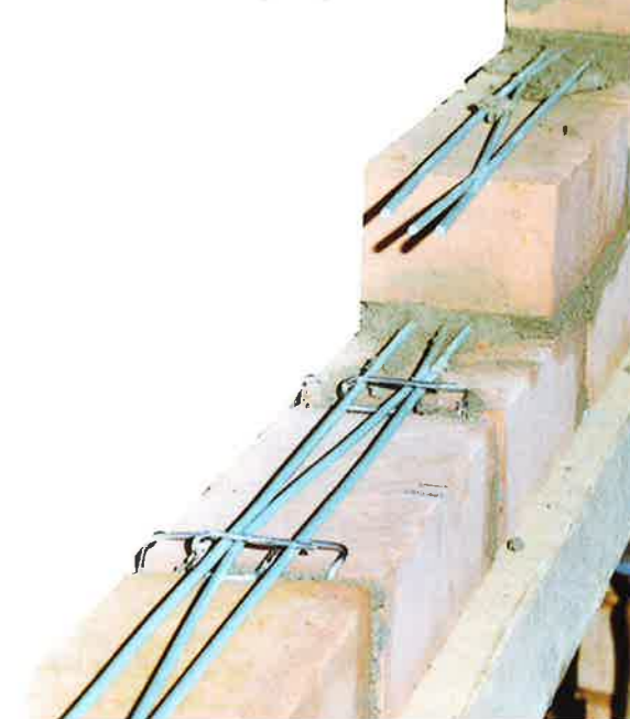
Inmetselen metselwerkwapening
